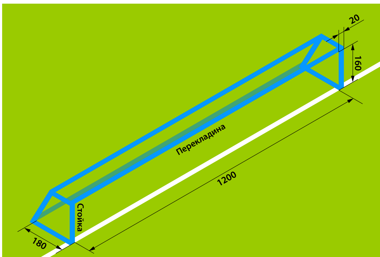
Рис. 3. Схема ворот
